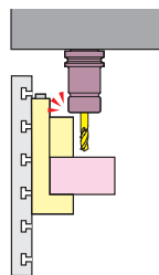
ホルダとバイスが干渉する
